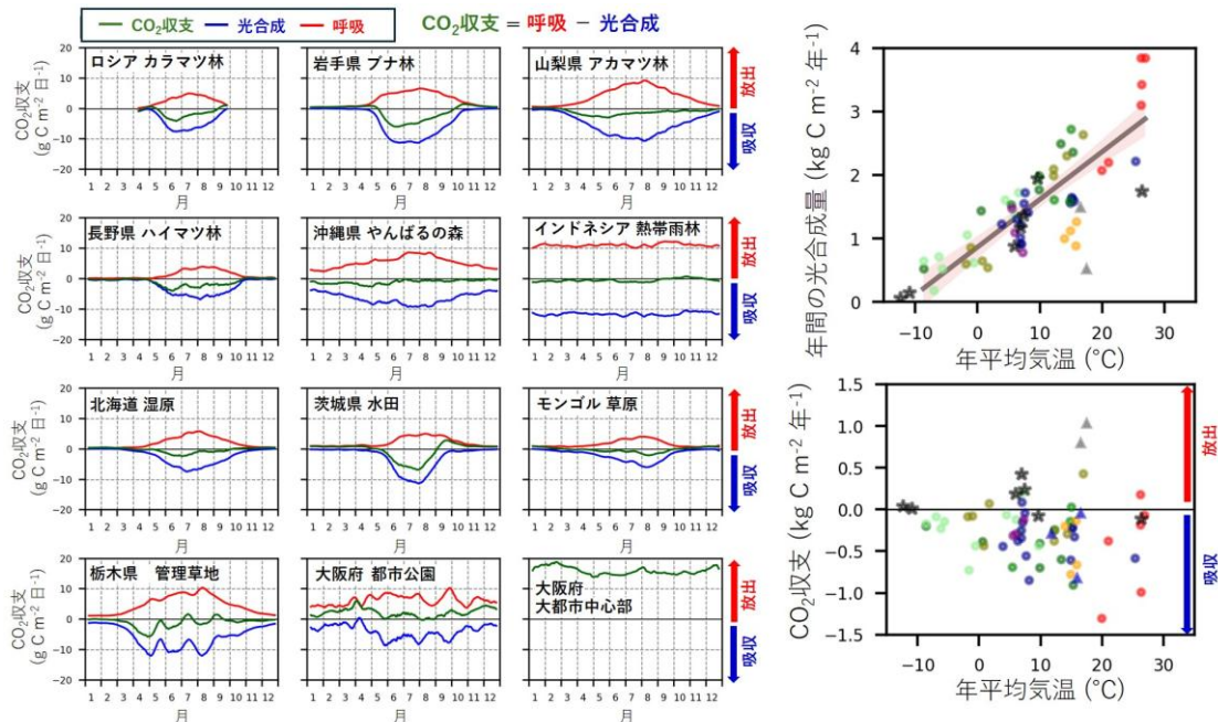
図3 いくつかの生態系・都市を対象としたCO 2 収支の平均的な季節変化パターン CO 2 収支および年間の光合成量を示したグラフにおけるシンボルの違いは、異なる生態系タイプを示す。
