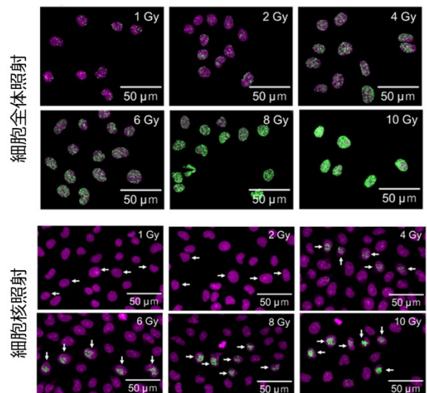
図 3 ハムスター細胞の全体を照射した場合（上）と細胞核を照射した場合（下、矢印は照射した細胞）の \gamma -H2AX フォーカス形成（ヒト細胞でも同様の結果が得られました）
