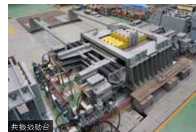
共振振動台
