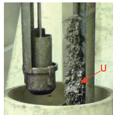
図4 使用済MOX燃料から回収したウラン 左側のルツボのMOX還元物から、右側の鉄棒にUを回収。針状結晶が特徴。
