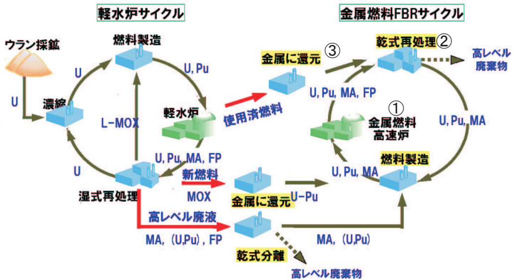
図1 原子燃料サイクルにおける金属燃料サイクル 軽水炉サイクルと高速炉サイクルが乾式再処理により有機的につながったことが特徴。 ①、②、③は主な成果1、2、3にそれぞれ対応する技術を示す。
