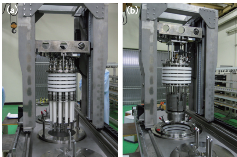
図3 開発した乾式再処理の工学規模試験装置 (a) 酸化物燃料を金属に還元する装置 (b) 還元した金属燃料から U を回収する電解精製装置 本装置により、工学ホット試験に向け、スケールアップと処理速度、信頼性の向上を実証することが可能となった。
