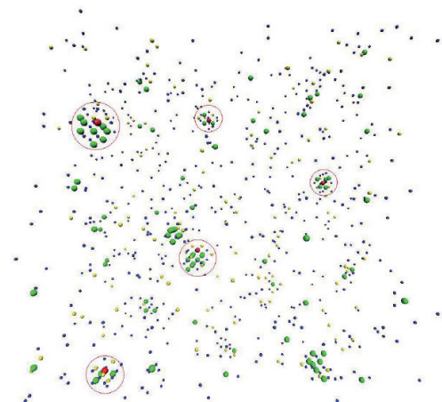
図3 原子空孔（赤）の拡散による溶質原子（緑：Cu、青：Ni、黄：Si）クラスターの形成 原子空孔を核にクラスターが形成されている。
