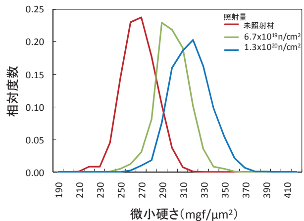
図5 中性子照射された压力容器鋼の硬さ分布分布を比較することで、僅かな硬さの変化を正確に測定可能することができる。
