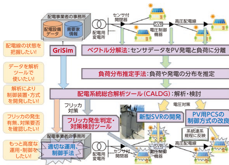
開発した配電システムの検討ツールの概要
